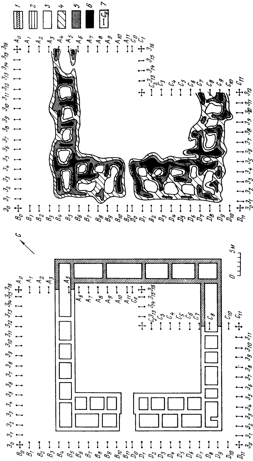
Рис. 2. Результаты электропрофилирования методом среднего градиента
