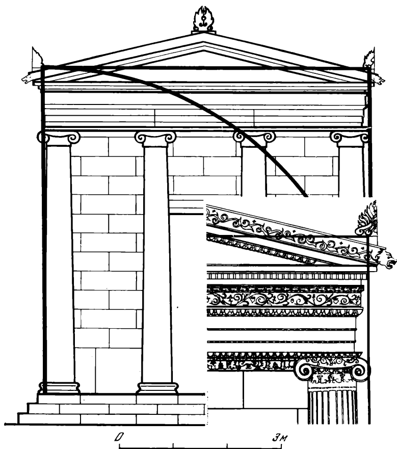
Рис. 3. Фасад ионического простиля. Херсонес. Реконструкция автора
