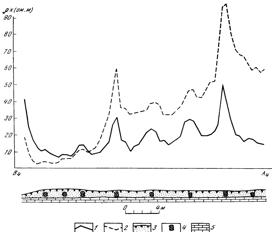
Рис. 1. Графики электропрофилирования и схематический разрез усадьбы 1 — график \rho_k симметричного электропрофилирования; 2 — график \rho_k срединного градиента; 3 — дневная поверхность и отложения культурного слоя; 4 — доколи стен усадьбы; 5 — материк (известняк)
