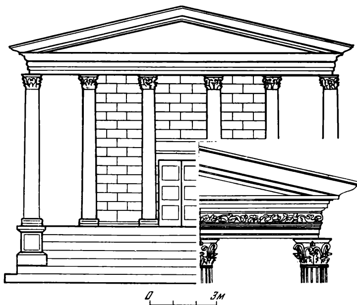
Рис. 5. Фасад коринфского периптера. Горгишья. Реконструкция автора
