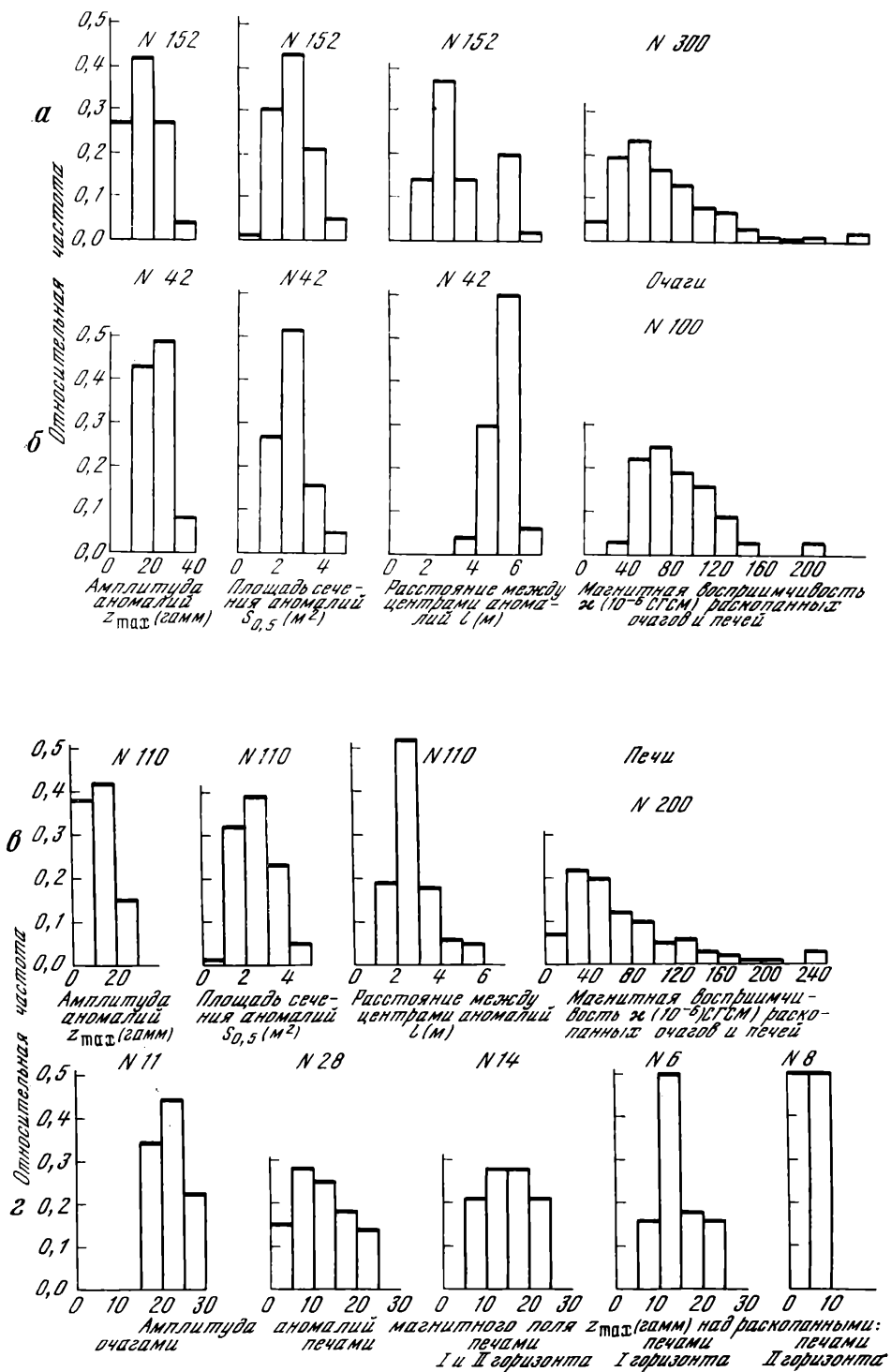
Рис. 3. Гистограммы характеристик аномалий магнитного поля: а) генеральной совокупности аномалий; б) совокупностей аномалий центральных и периферийных рядов; в) совокупности аномалий остальных рядов; г) аномалий над раскопанными объектами
