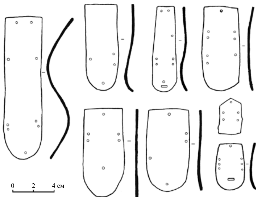
Рис. 92. Пластины ламеллярного панциря из ст. Тбилисской, 15/1
