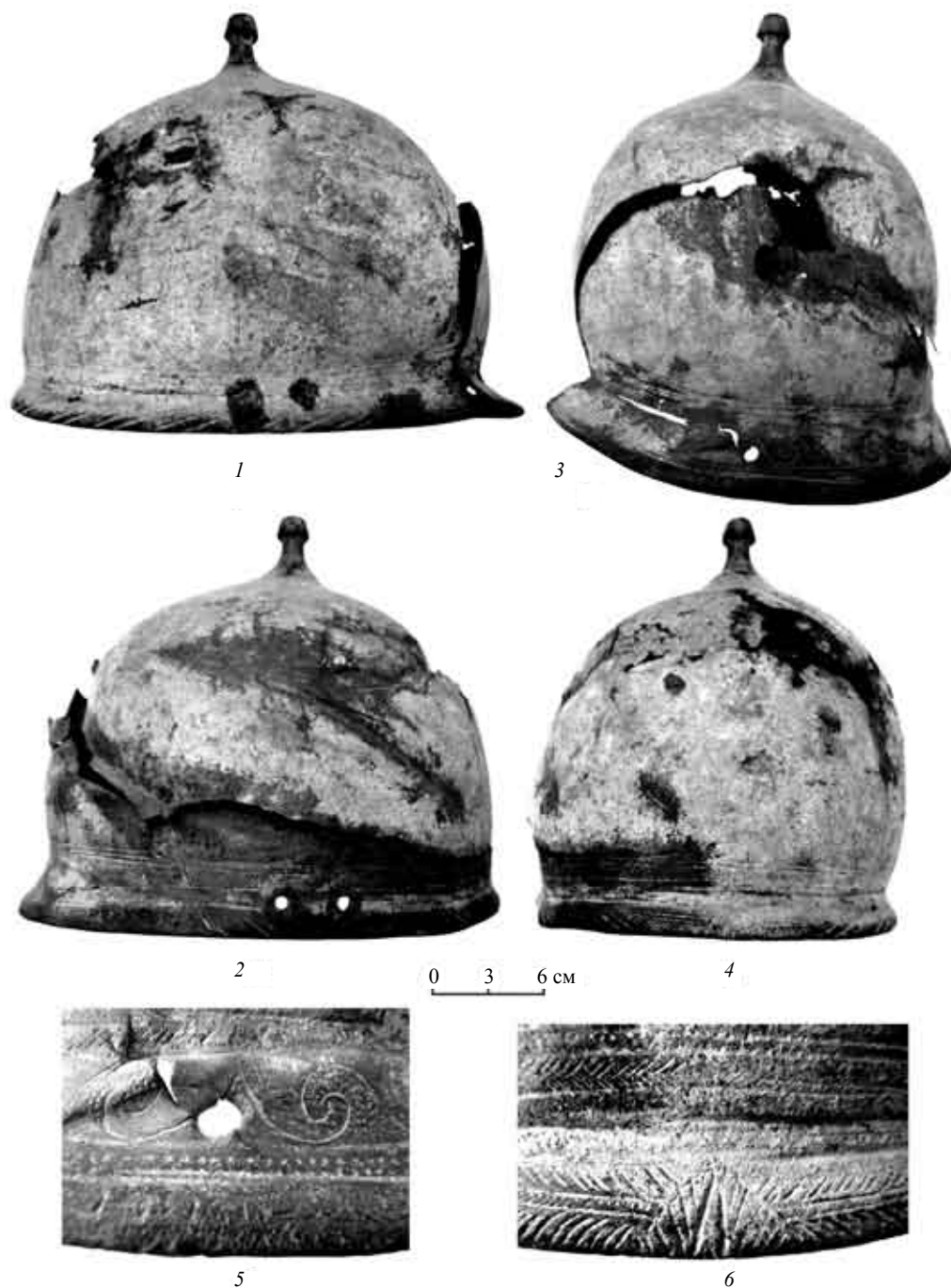
Рис. 113. Шлем из Беленького: 1, 2 — вид сбоку; 3 — вид сзади; 4 — вид спереди; 5 — назатыльник (деталь); 6 — фронтальная часть (деталь)
