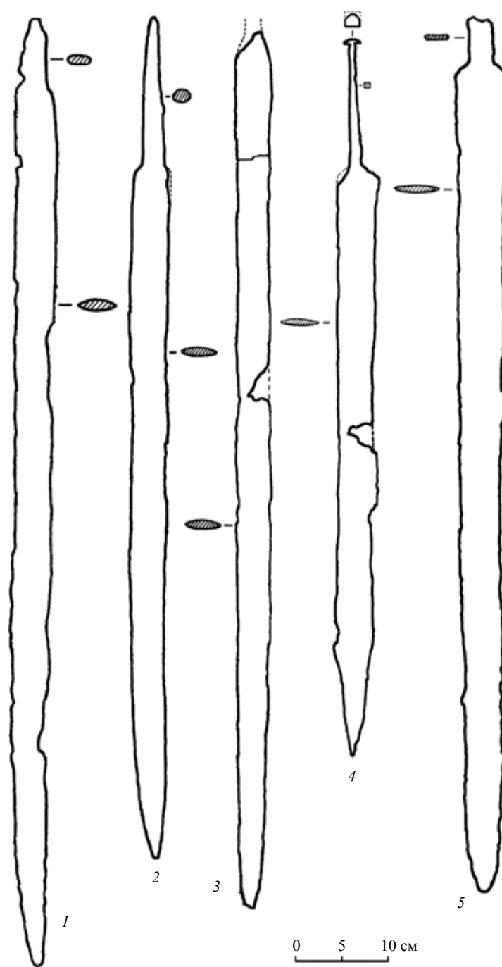
Рис. 28. Мечи с рукоятью-штырем 2-го типа: 1 — Маяки; 2 — Усть-Каменка, 37/1; 3 — Усть-Каменка, 40/1; 4 — Водославка; 5 — Светловодск
