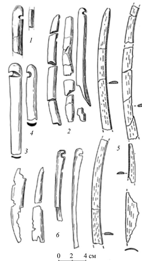
Рис. 66. Костяные накладки на лук из сарматских погребений: 1 — ст. Усть-Лабинская, 29/1 (Гущина, Засецкая, 1994); 2 — Суслы, 51/1 (Хазанов, 1971); 3 — Калиновка, 36/1; 4 — Калиновка, 7/1 (Шилов, 1959); 5 — Центральный VI, 16/8 (Безуглов, 1988); 6 — Нижний Баскунчак, 2 (Хазанов, 1971)
