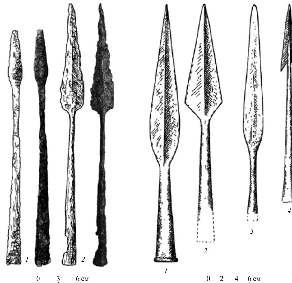
Рис. 45. Наконечники копий типа 1: 1 — Квашино; 2 — Великоплатное
