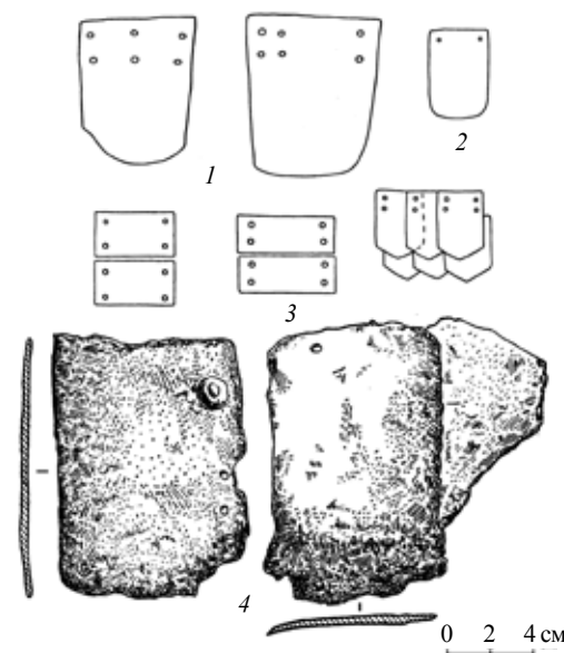
Рис. 73. Чешуйки сарматских панцирей:
