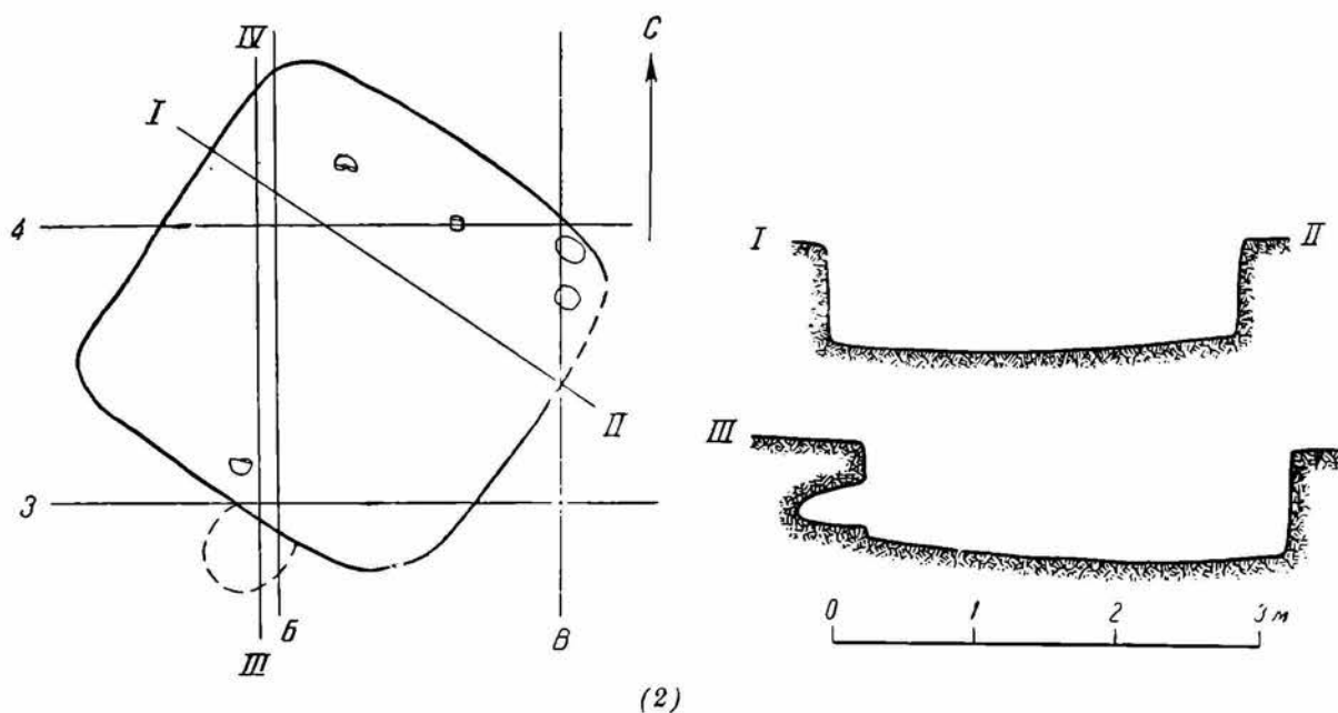
Рис. 7. Поселение у с. Битицы. Общий вид (1), план и разрезы к нему (2) постройки № 1.
