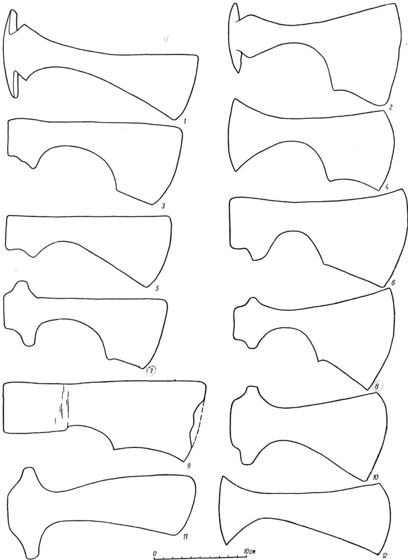
Табл. XVI. Рабочие топоры X-XIII вв.
