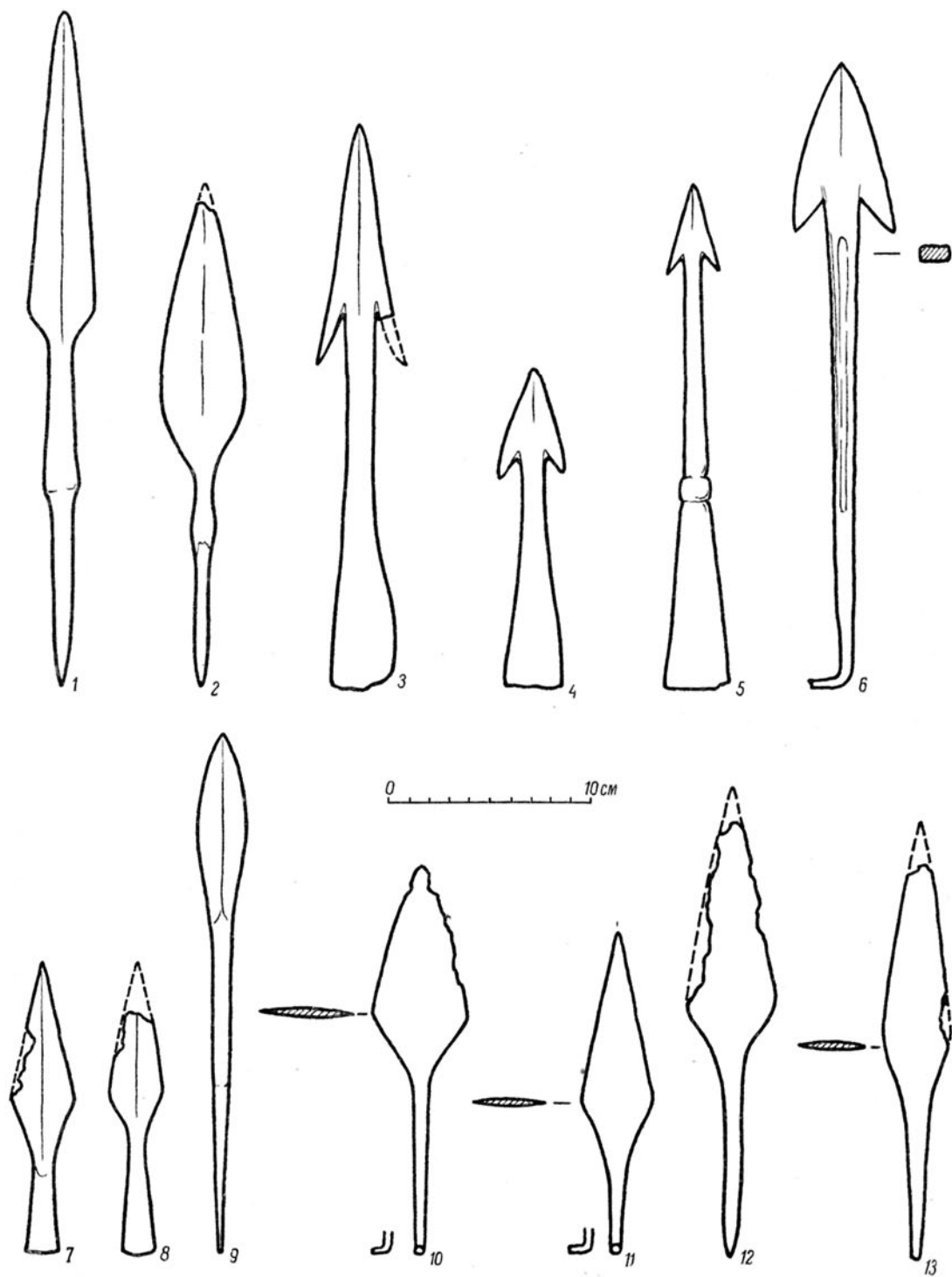
Табл. X. Копья (1—6) и сулицы (7—13) X—XIII вв.
