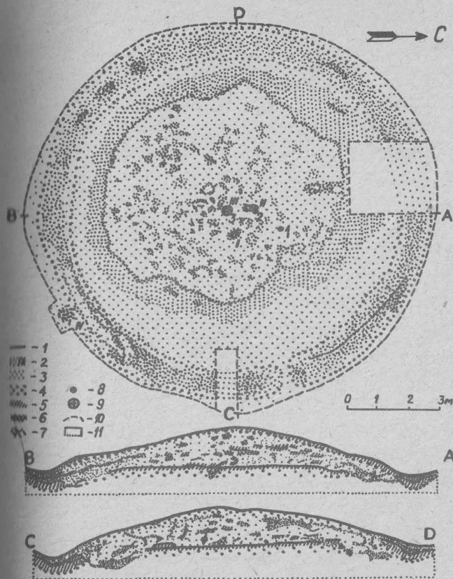
Рис. 15. Сводный план кургана 9 в Лаоссина II.
